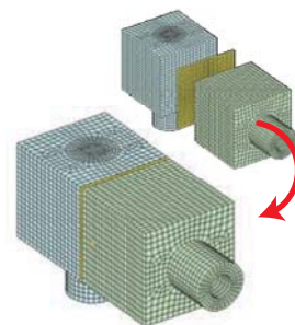
事例2 節点の不連続なモデルの解析
