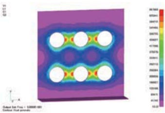
温度分布 (PHOTO-THERMOによる)
