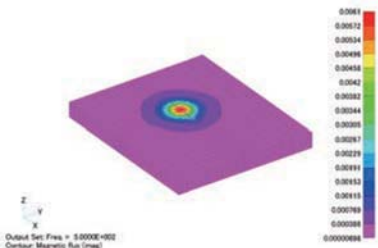
解析結果(磁場コンタ図)
