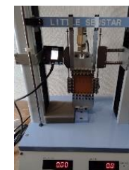
二軸引張試験
